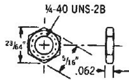
Std. Hex Nut
